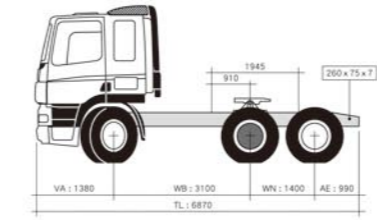
FTR CF85 460 6X2曳引車
