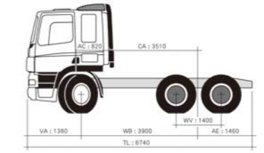
FTT CF85 460 6X4曳引車
