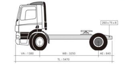
FT CF85 360/410 4x2曳引車
