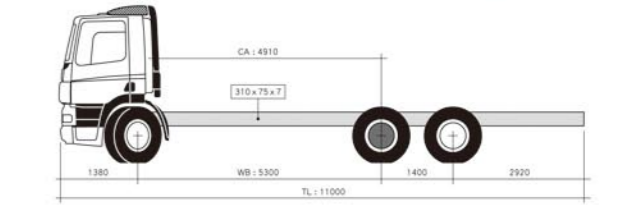
FAR CF85 410 6x2兼供曳引用的大貨車(全拖)
