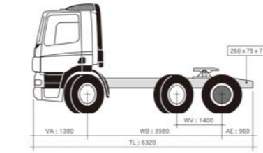
FTG CF85 410 6X2曳引車
